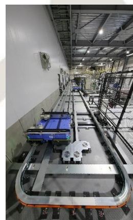
自動搬送台車
